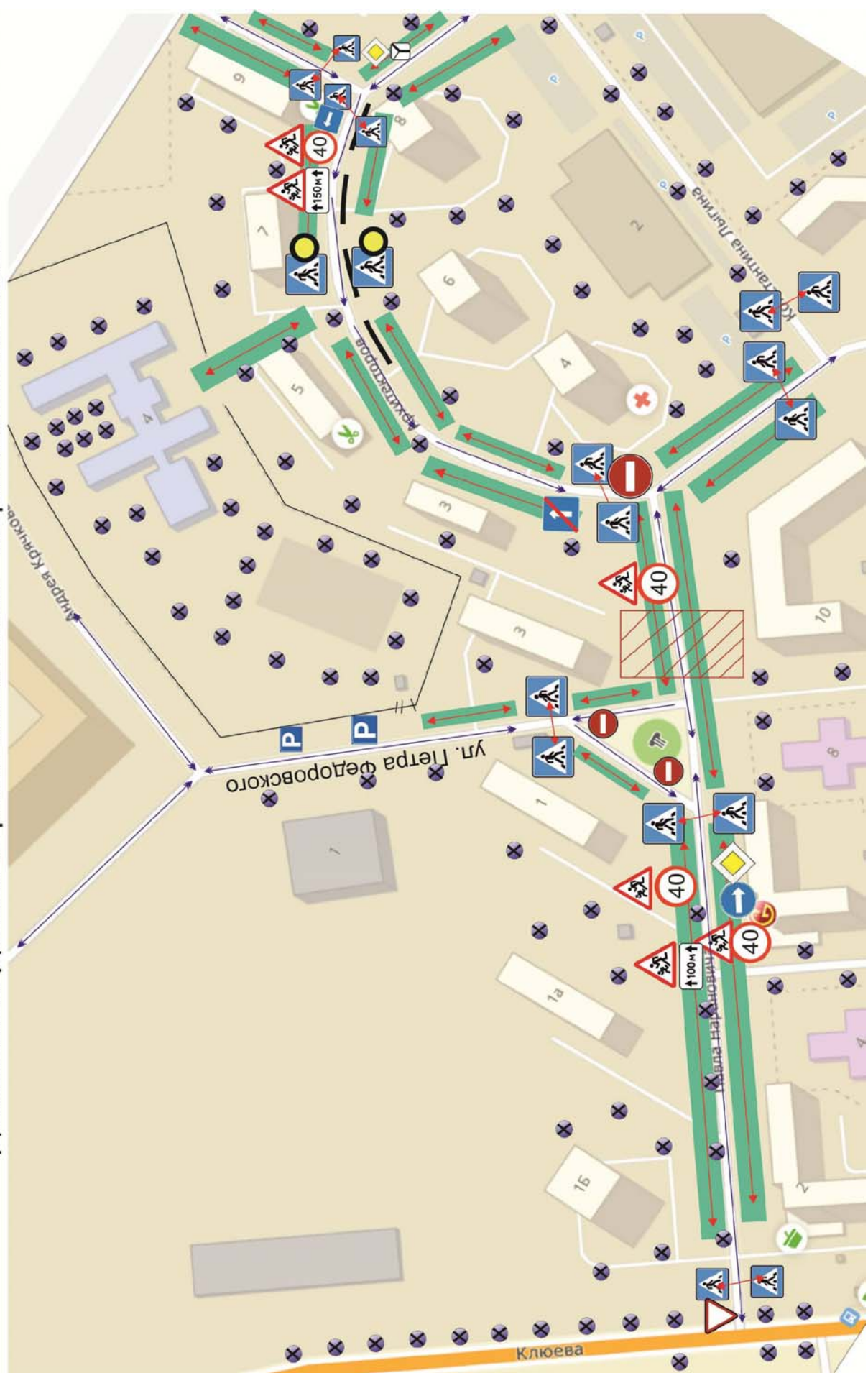
2. Схема организации дорожного движения в непосредственной близости от образовательного учреждения с размещением соответствующих технических средств организации дорожного движения, маршрутов движения детей и расположении парковочных мест
